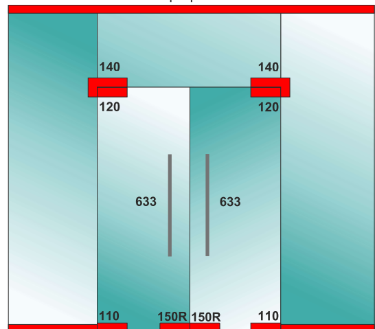
84D Схема №12
